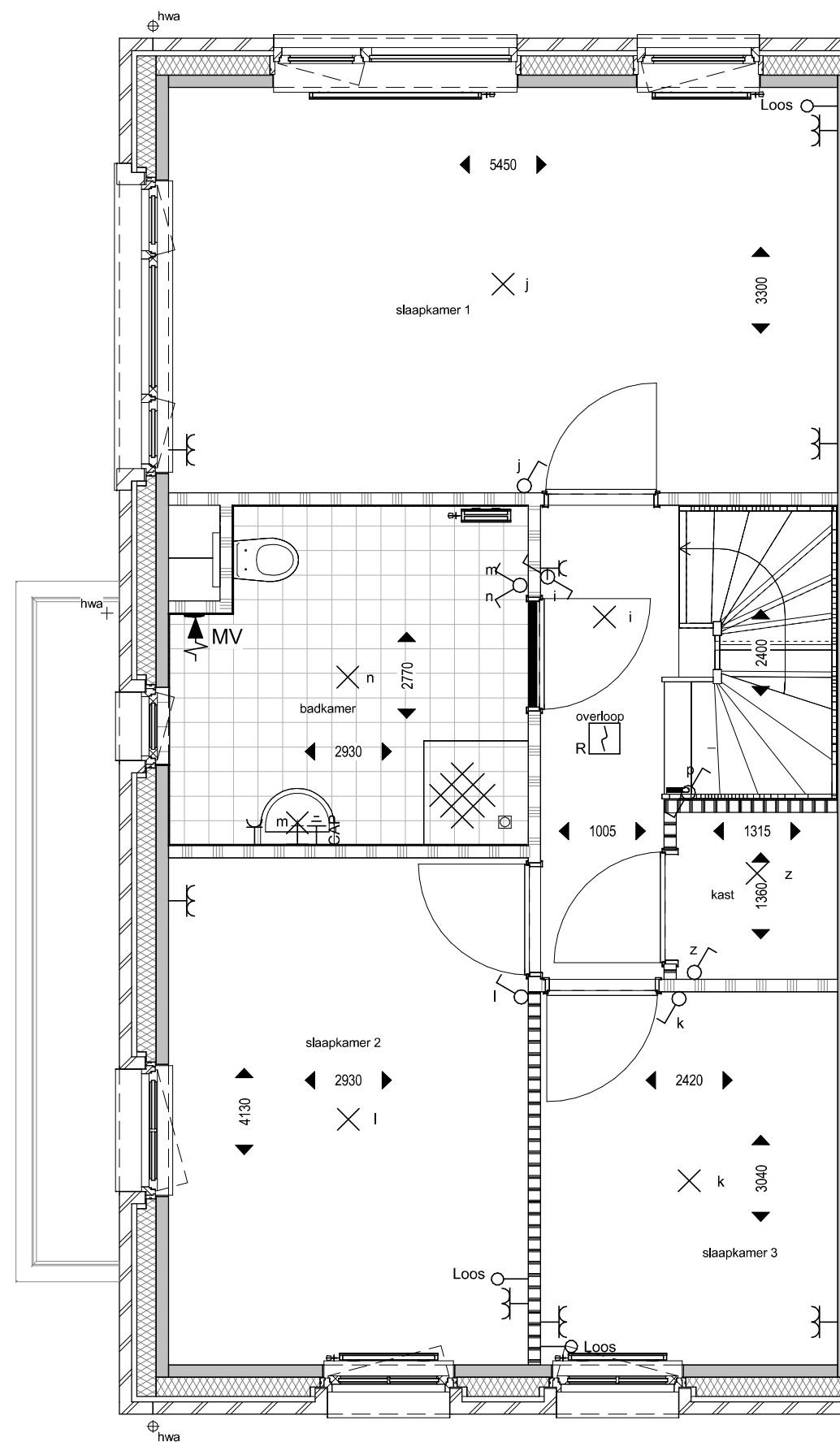
Eerste verdieping
